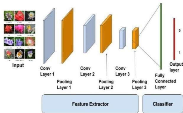
Fig 1 CNN
